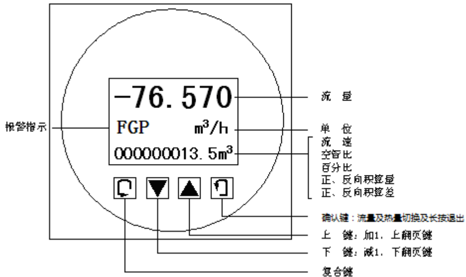
图 4.3 键盘定义与液晶显示（流量界面）
